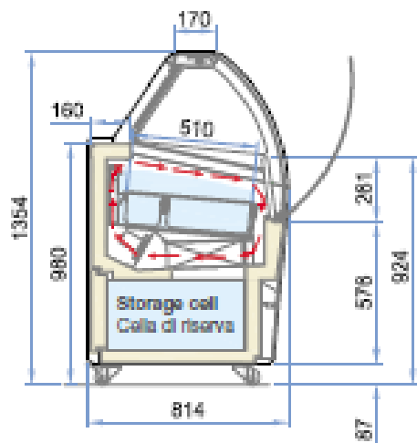
Wymiary rysunek
